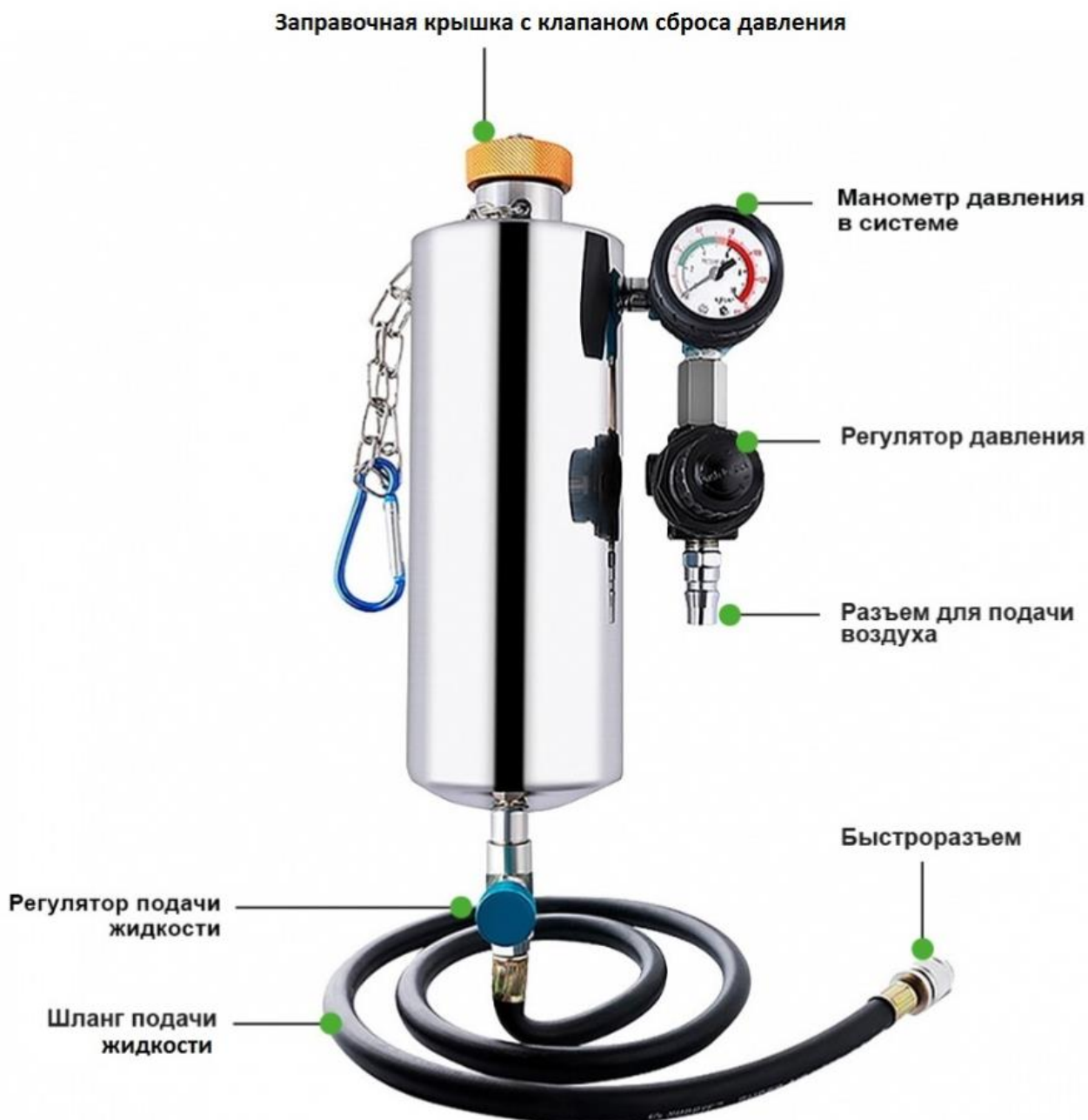
Рис.2 Устройство аппарата GX-100
